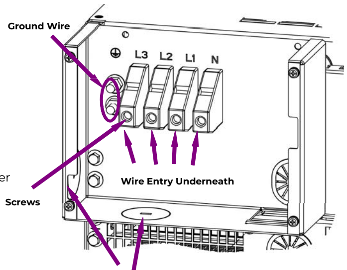
AC conduit connection knockouts for 1" conduit
