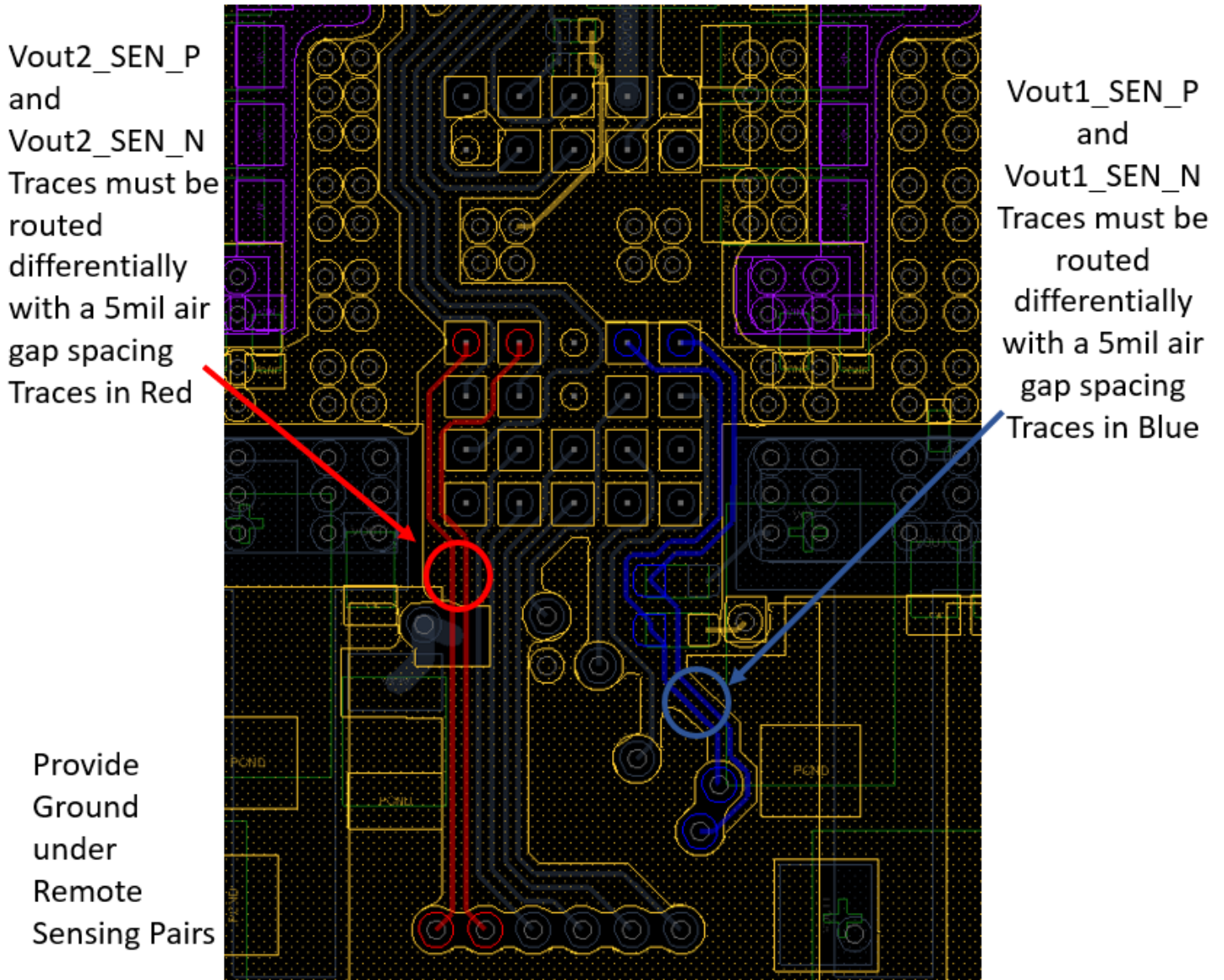
Figure 33 : VSense Traces
