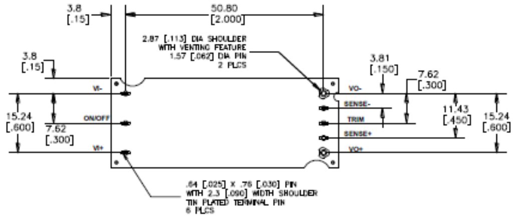
Bottom View*
