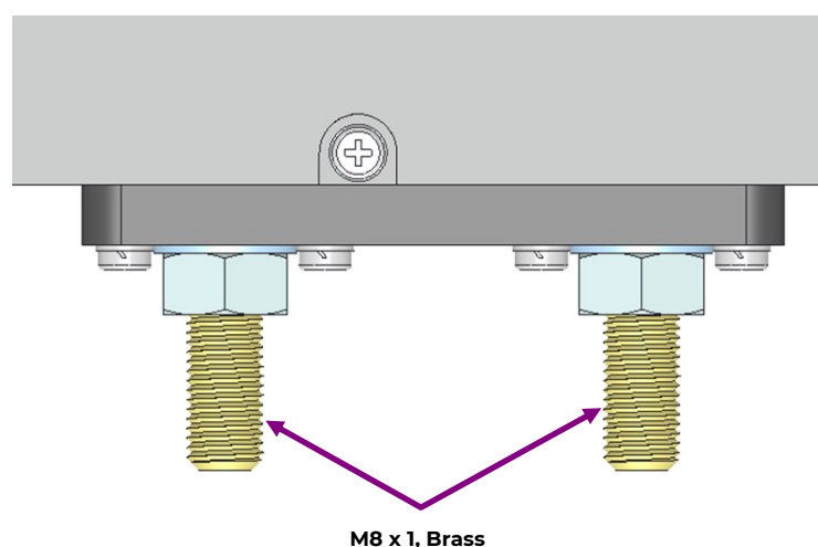
Rectifier output connectors
